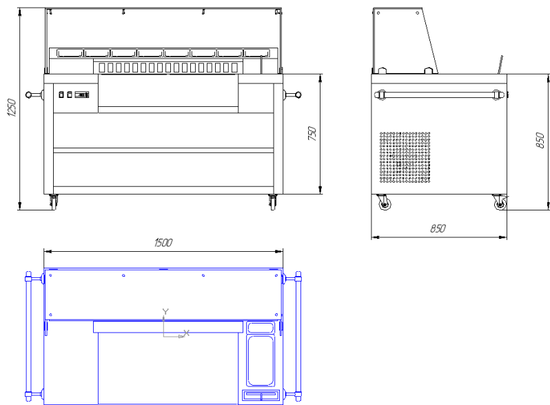
Рис. 1 Блинная станция с охлаждаемой ванной
